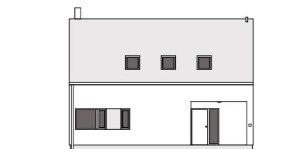
POHLED P1
