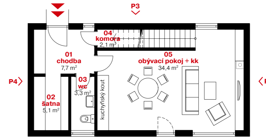
PŮDORYS PŘÍZEMÍ
