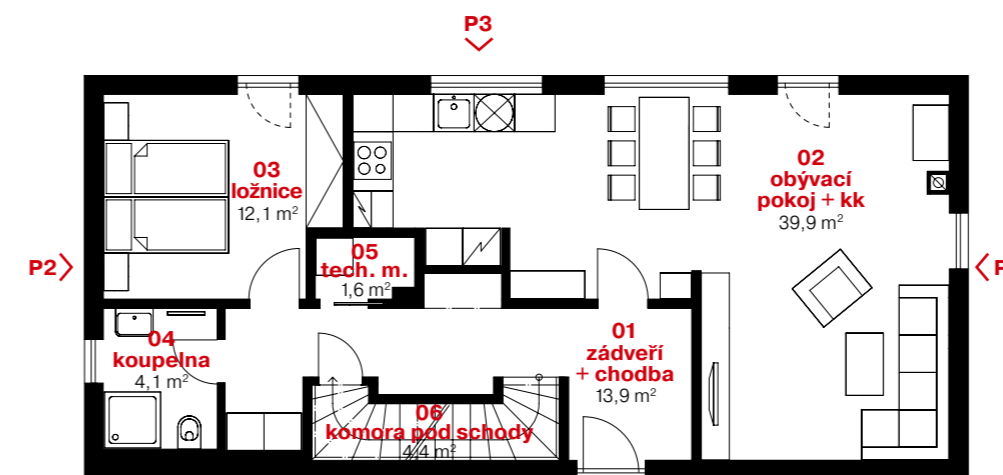
PŮDORYS PŘÍZEMÍ
