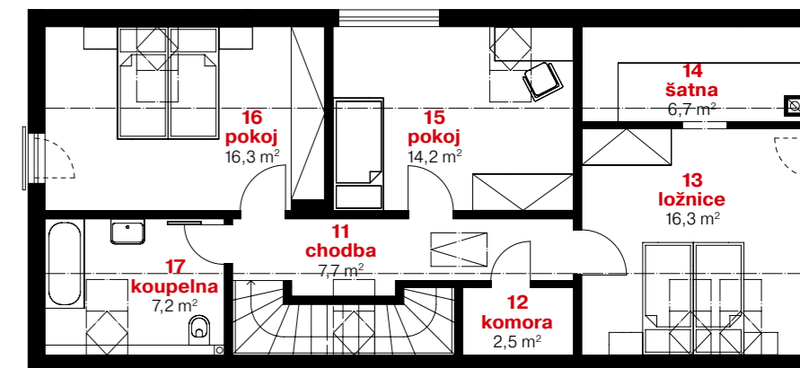
PŮDORYS PATRA
