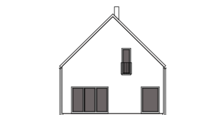
POHLED P4
